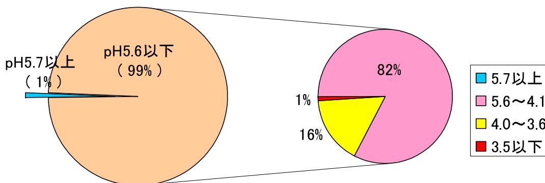
図 1-1 全降雨に占める酸性雨の割合
