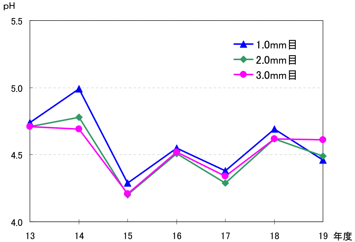
図7 初期降雨のpH経年変化(さいたま市役所測定局)
