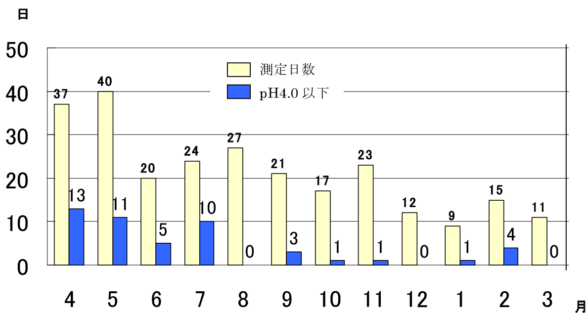
図4 pH4.0以下の降雨日数経月変化
