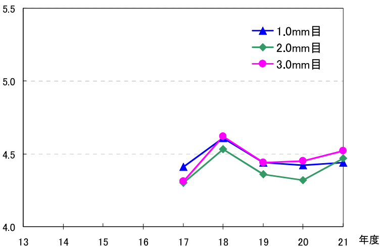
図4-5 初期降雨のpH経年変化(岩槻測定局)
