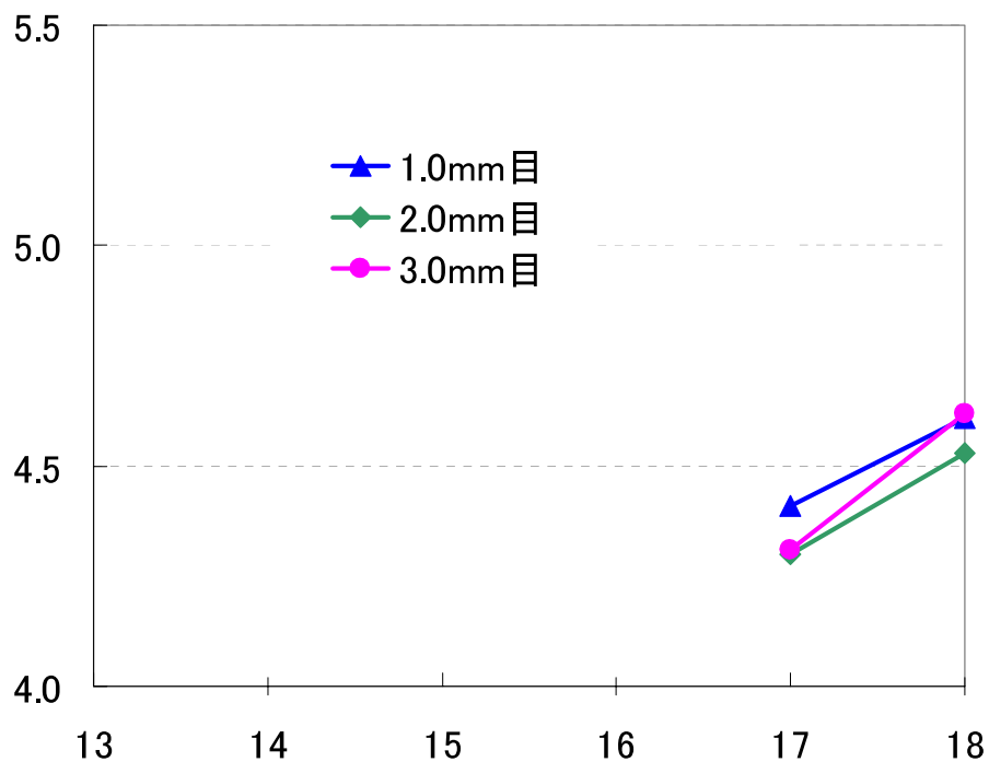
図 1 1 初期降雨の pH 経年変化 (岩槻測定局)
