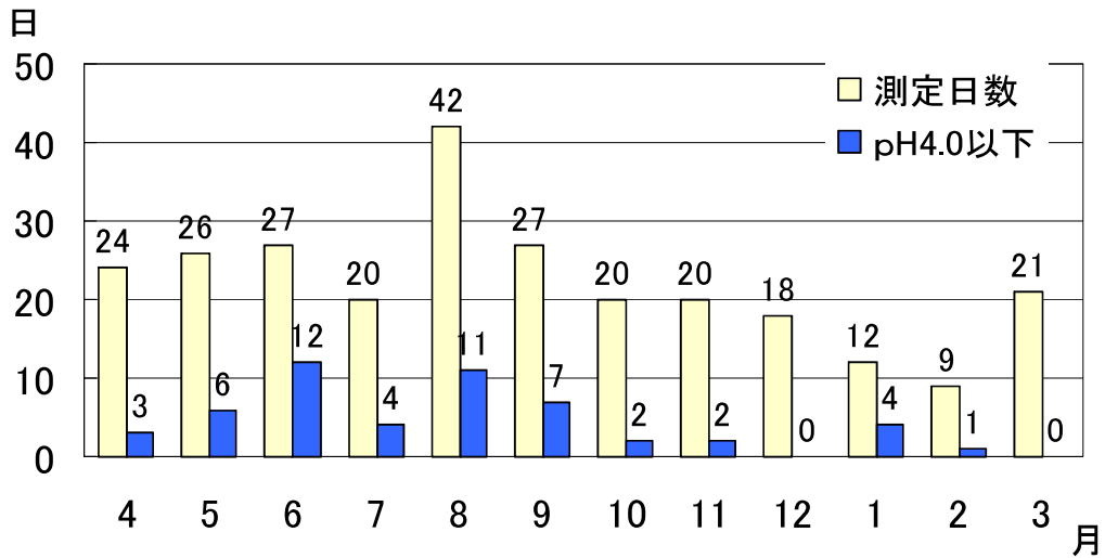
図2 pH4.0以下の降雨日数経月変化(3局合計)
