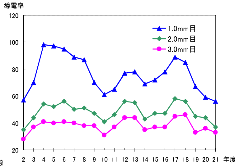
図4-4 初期降雨の導電率経年変化(大宮区役所)
