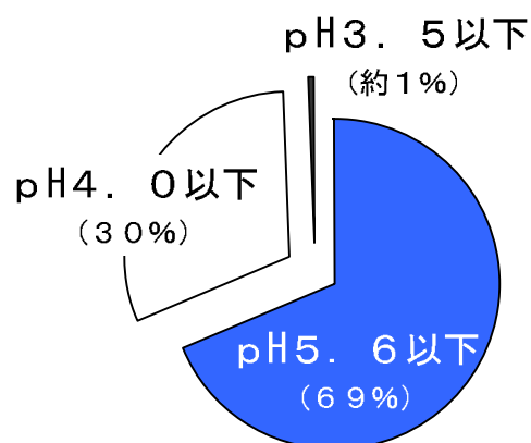
図3 酸性雨中の酸性度分布
