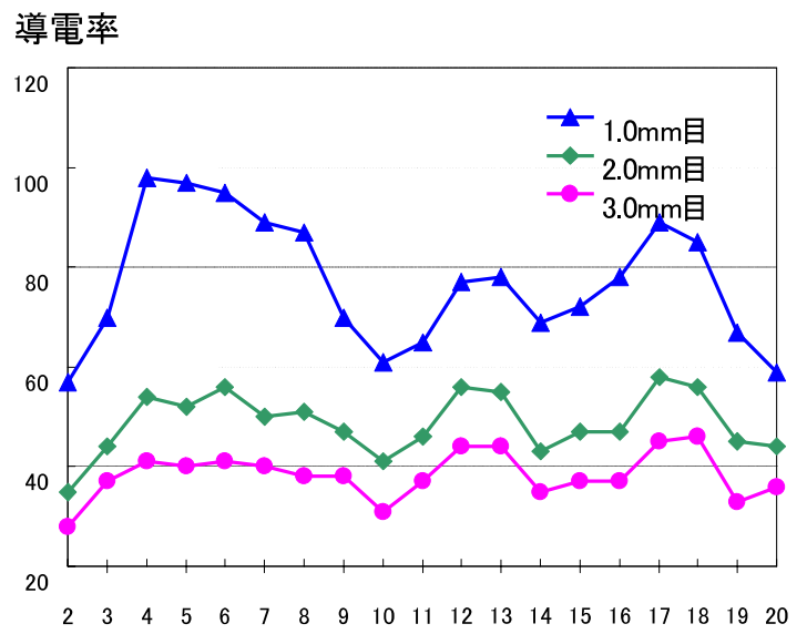
図 4-4 初期降雨の導電率経年変化(大宮区役所)
