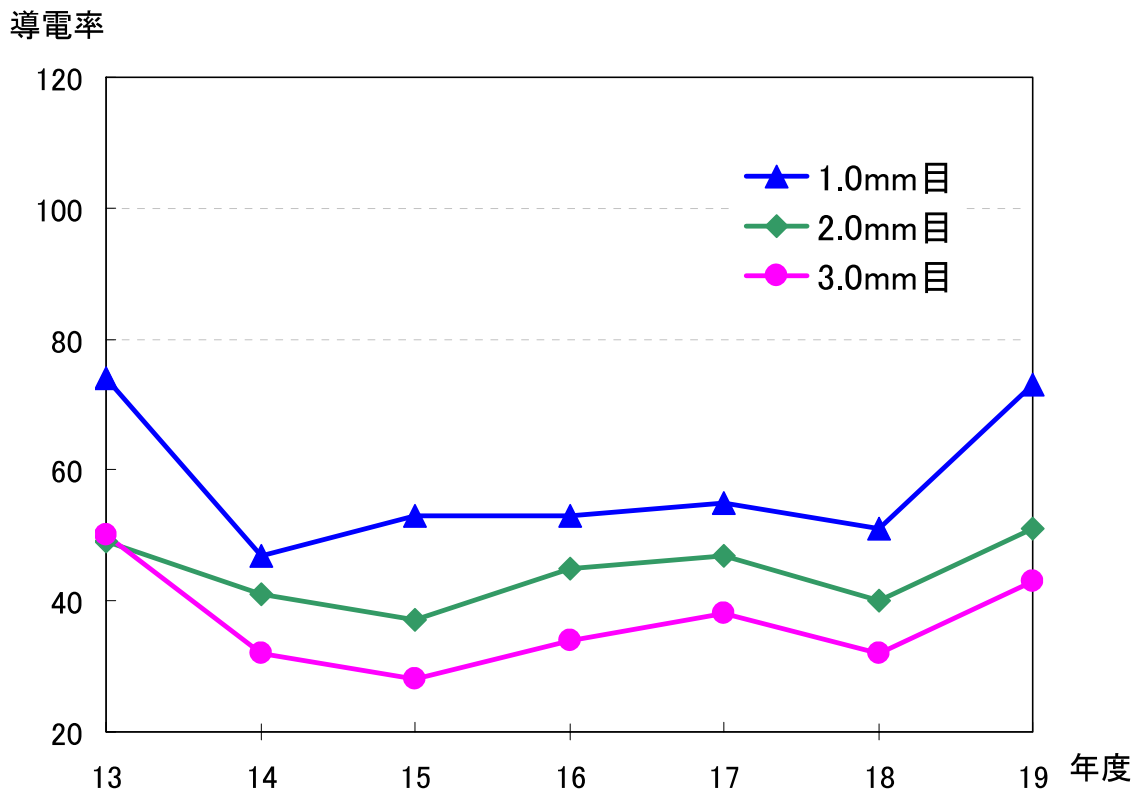
図8 初期降雨の導電率経年変化(さいたま市役所測定局)
