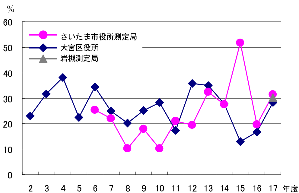
図5 全降雨日数に占める酸性雨（pH4.0以下）の割合の経年変化
