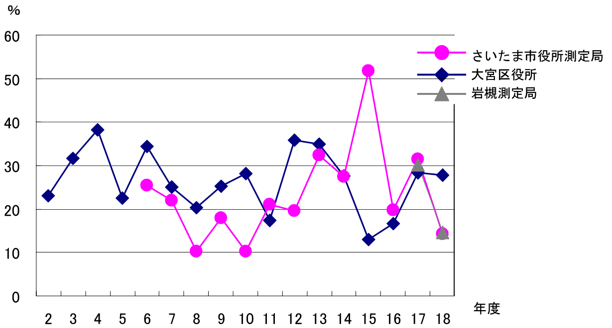
図5 全降雨日数に占める酸性雨 (pH4.0 以下) の割合の経年変化
