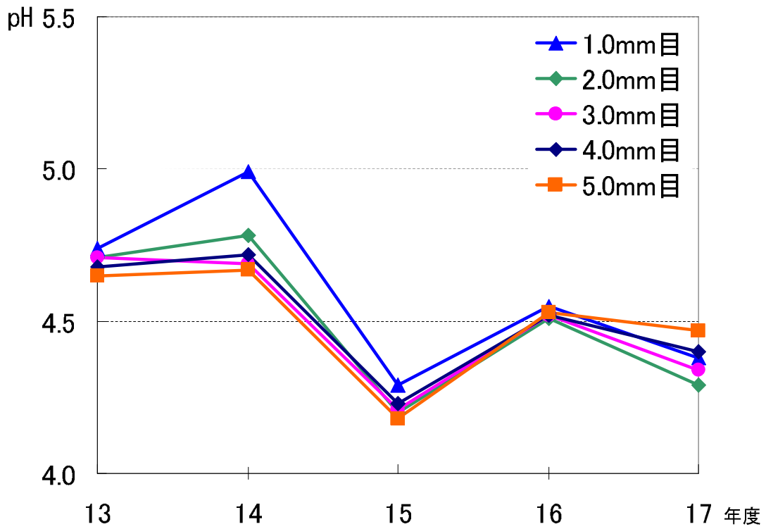
図6 初期降雨のpH経年変化(さいたま市役所測定局)
