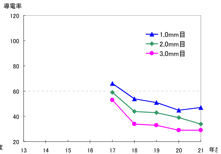
図4-6 初期降雨の導電率経年変化(岩槻測定局)
