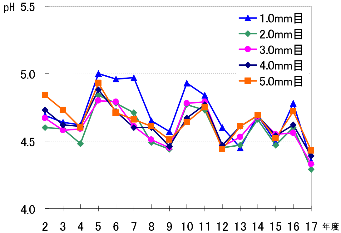
図8 初期降雨のpH経年変化（大宮区役所）
