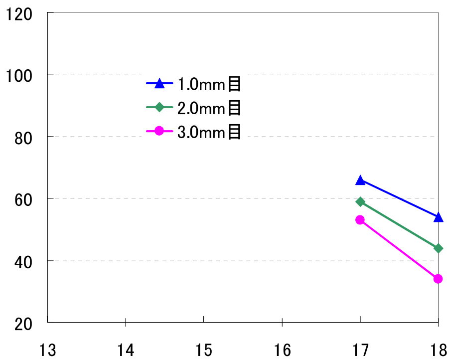
図 1 2 初期降雨の導電率経年変化 (岩槻測定局)
