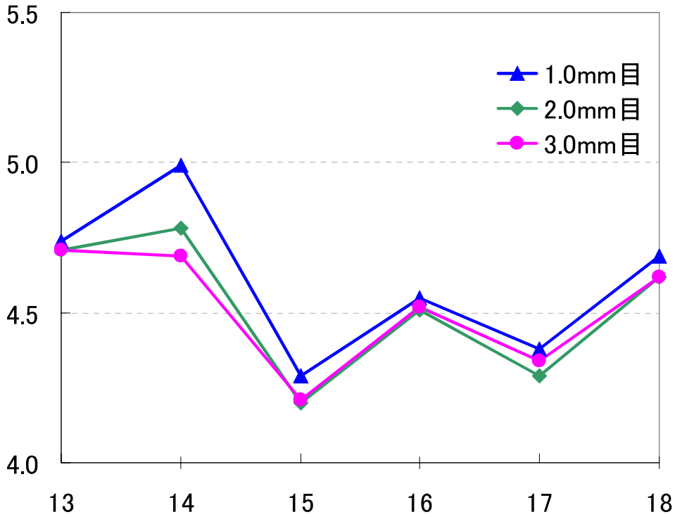
図7 初期降雨のpH経年変化 (さいたま市役所測定局)
