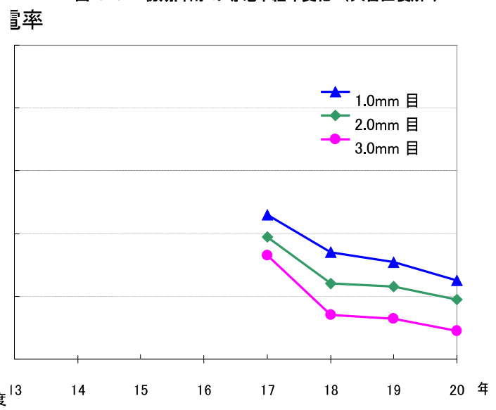
図 4-6 初期降雨の導電率経年変化(岩槻測定局)
