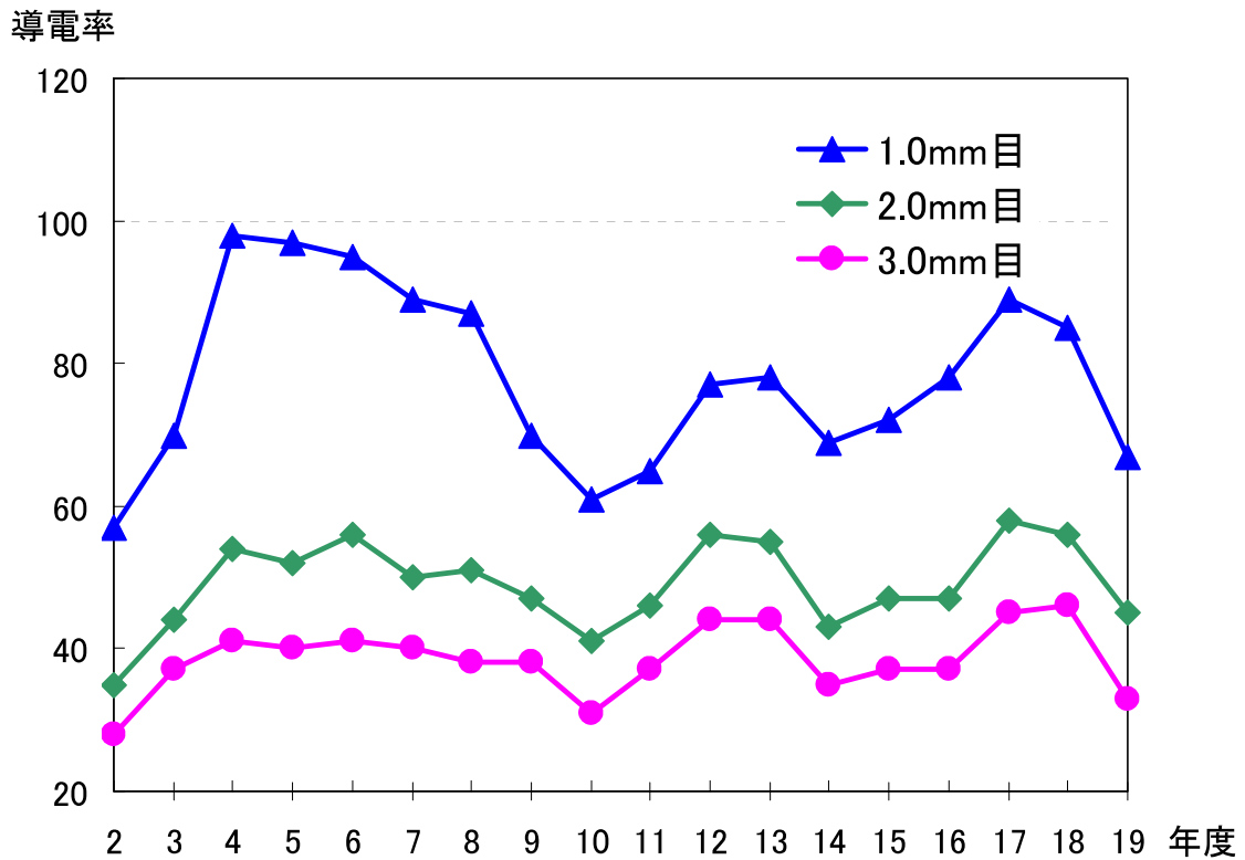
図10 初期降雨の導電率経年変化(大宮区役所)
