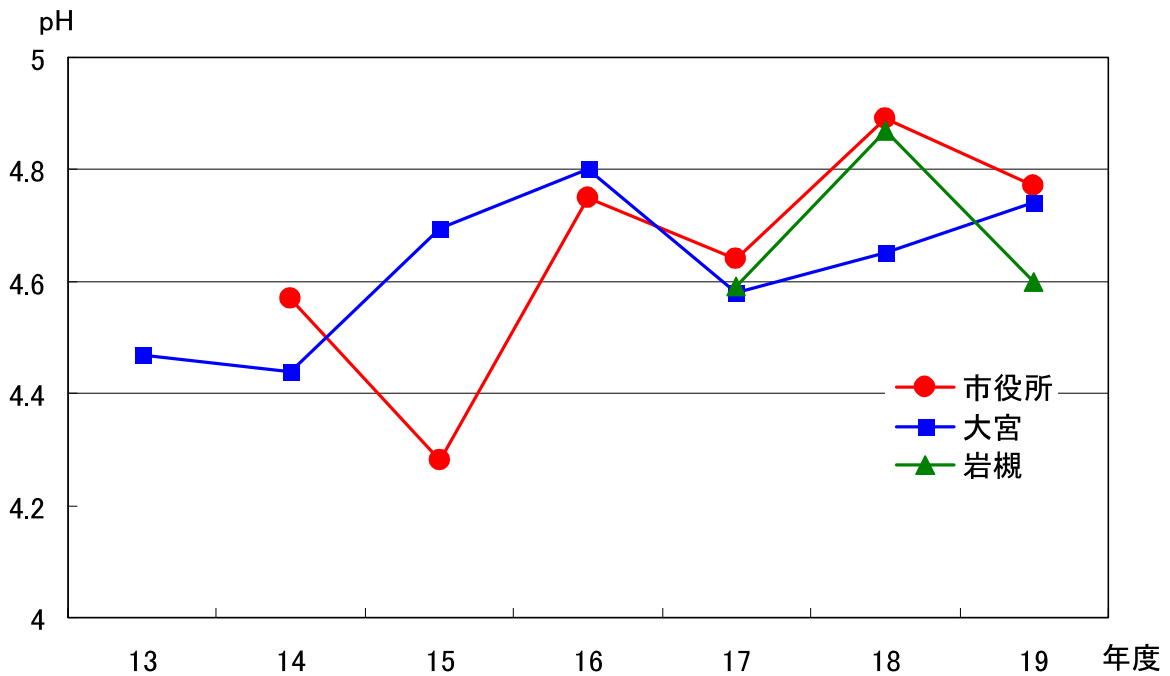
図6 年間平均pHの経年変化
