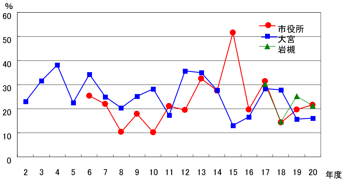
図3-2 全降雨日数に占める酸性雨(pH4.0以下)の割合の経年変化
