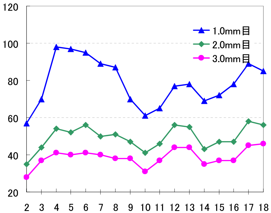
図10 初期降雨の導電率経年変化 (大宮区役所)
