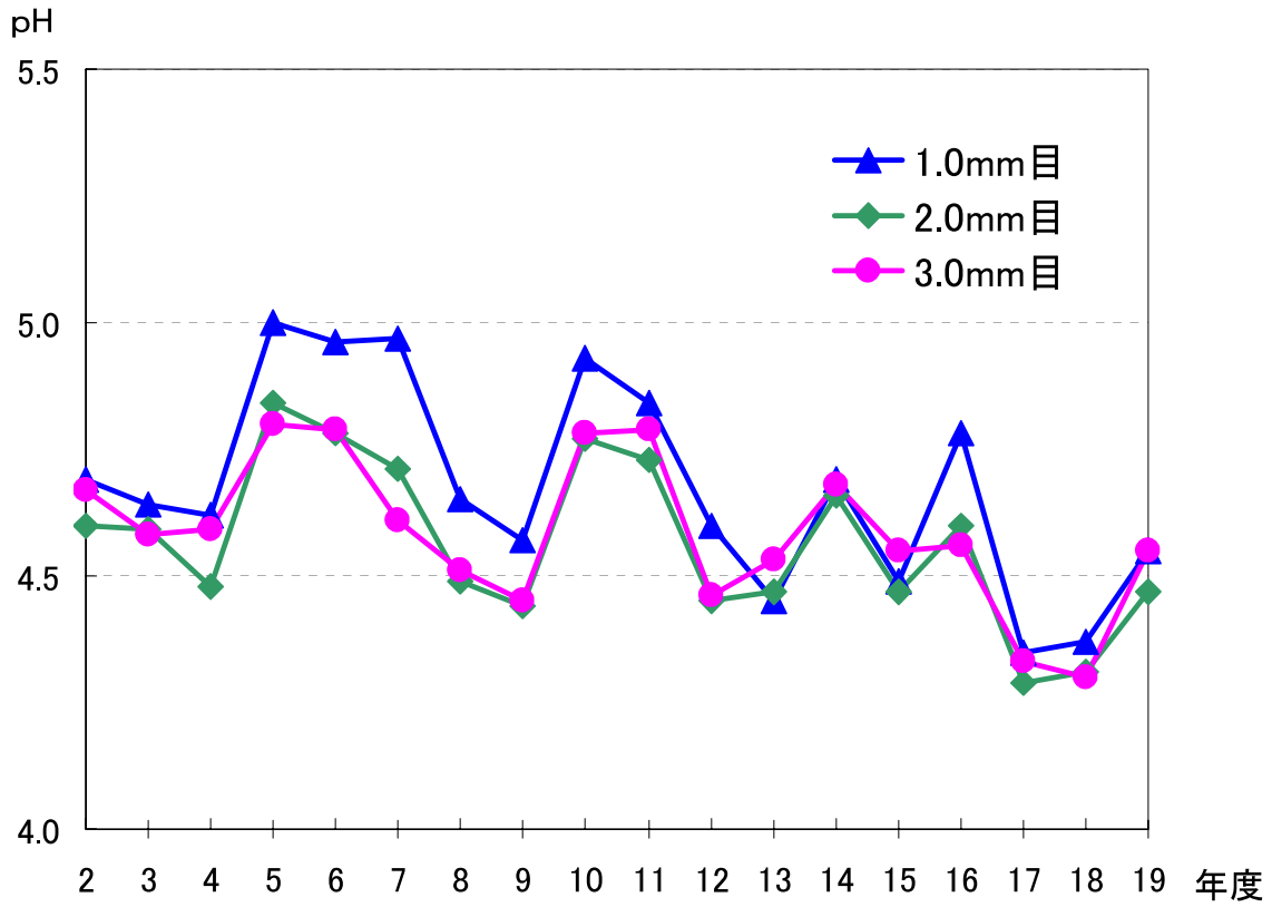
図9 初期降雨のpH経年変化(大宮区役所)
