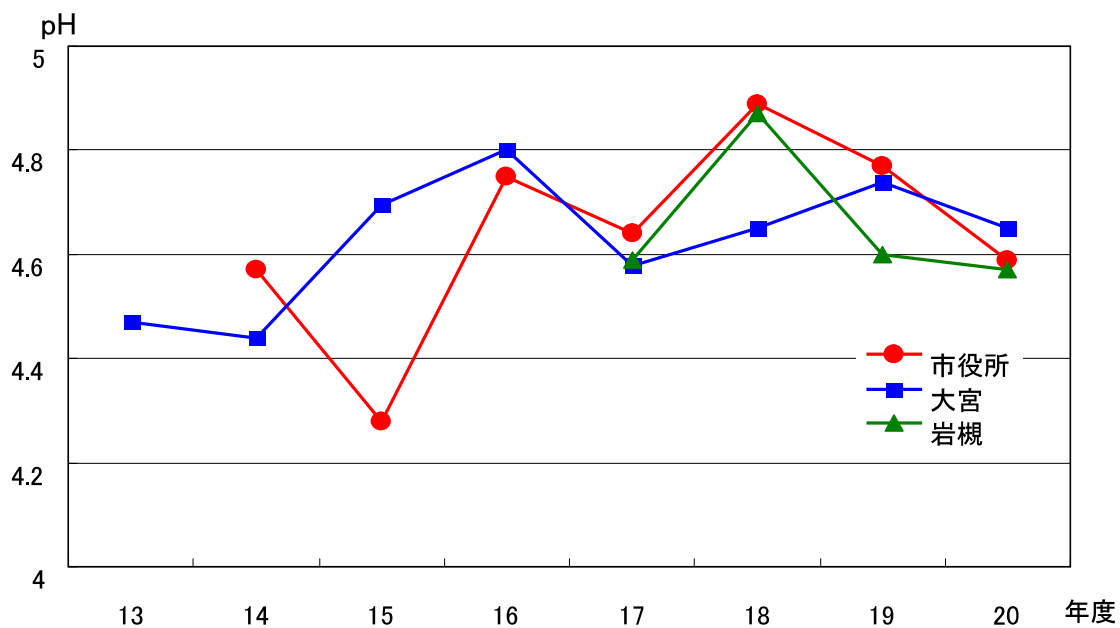
図 3-3 年間平均 pH の経年変化
