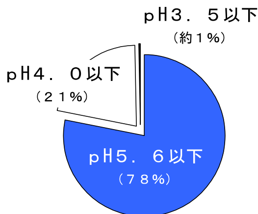
図 3 酸性雨中の酸性度分布
