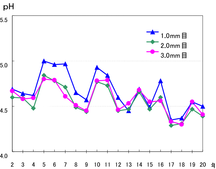
図 4-3 初期降雨のpH経年変化(大宮区役所)
