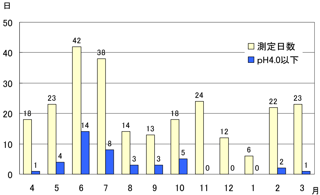
図2 pH4.0以下の降雨日数経月変化
