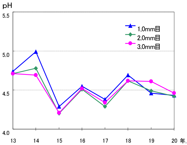
図 4-1 初期降雨のpH経年変化(さいたま市役所測定局)
