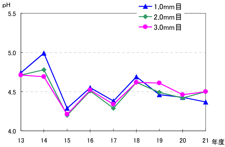
図4-1 初期降雨のpH経年変化(さいたま市役所測定局)
