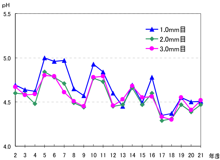
図4-3 初期降雨のpH経年変化(大宮区役所)
