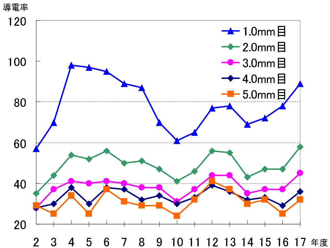
図9 初期降雨の導電率経年変化（大宮区役所）
