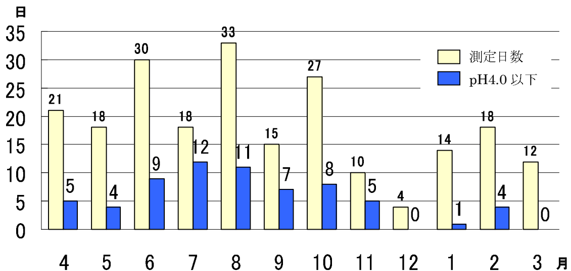
図4 pH4.0以下の降雨日数経月変化
