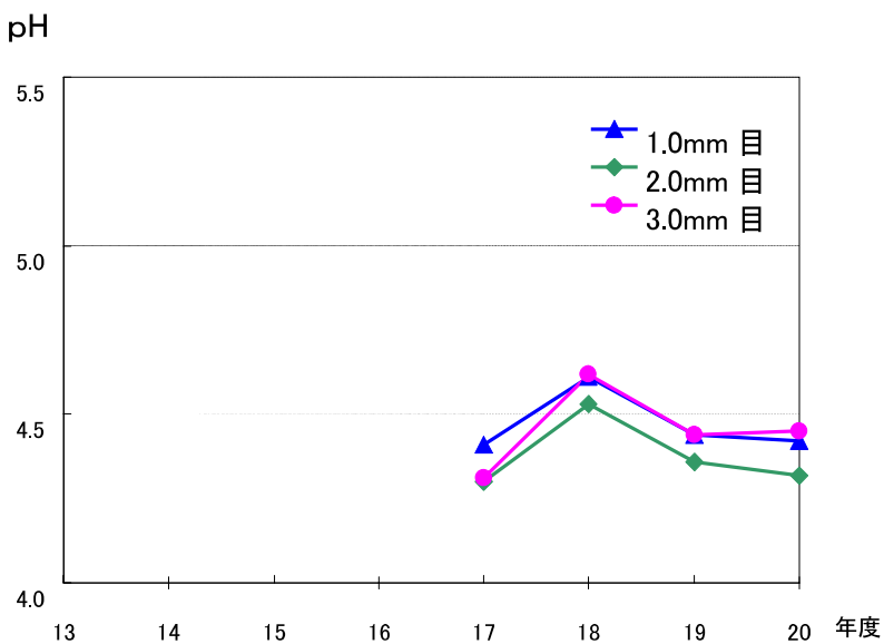
図 4-5 初期降雨のpH経年変化(岩槻測定局)
