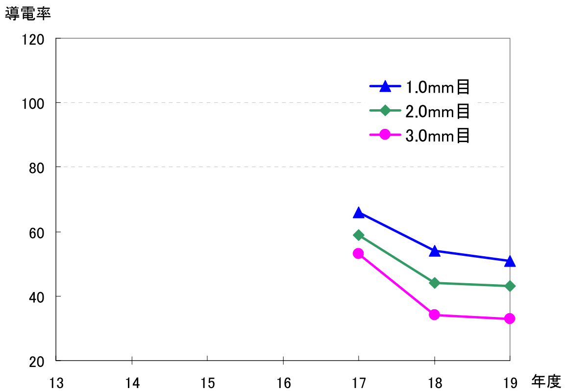
図12 初期降雨の導電率経年変化(岩槻測定局)
