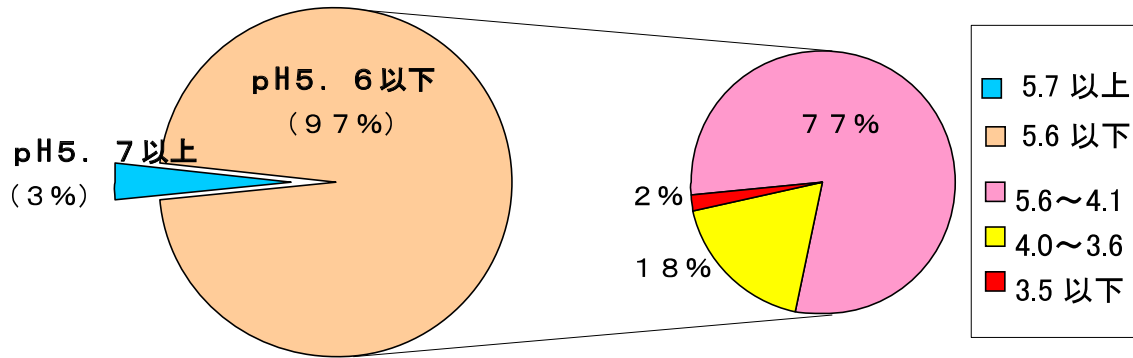
図 1-1 全降雨に占める酸性雨の割合
