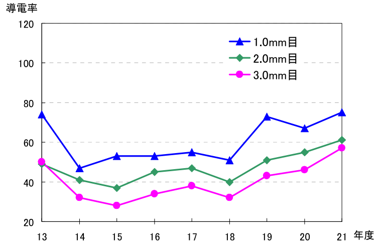
図4-2 初期降雨の導電率経年変化(さいたま市役所測定局)
