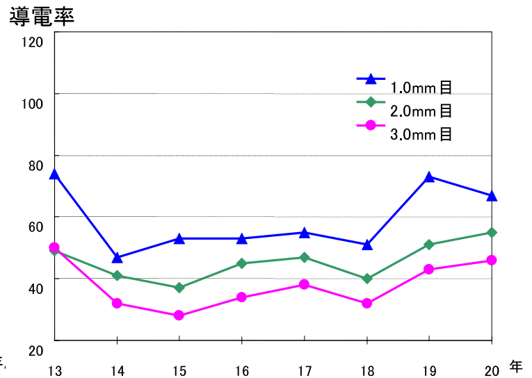
図 4-2 初期降雨の導電率経年変化(さいたま市役所測定局)
