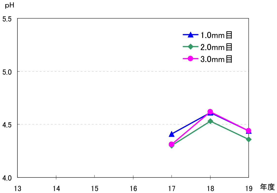
図11 初期降雨のpH経年変化(岩槻測定局)
