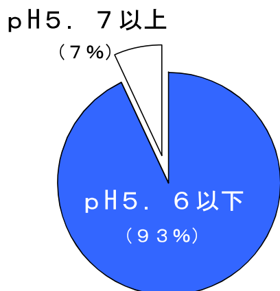
図 2 全降雨に占める酸性雨の割合
