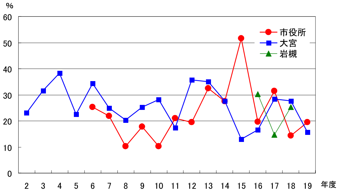
図5 全降雨日数に占める酸性雨(pH4.0以下)の割合の経年変化
