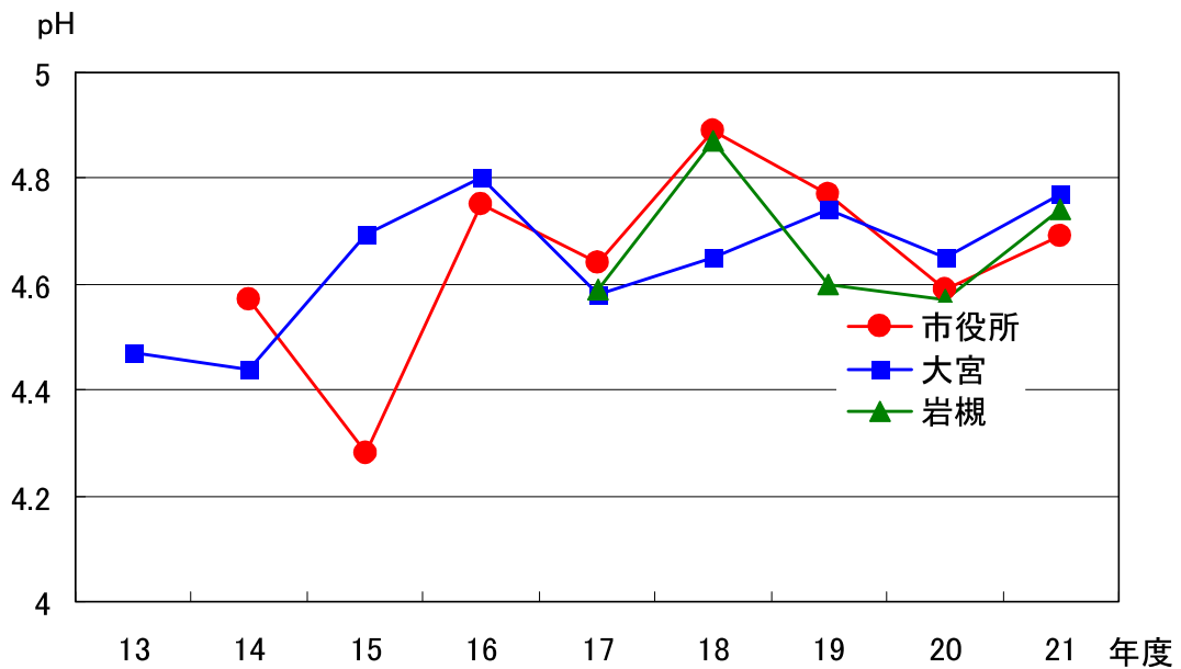
図3-3 年間平均pHの経年変化
