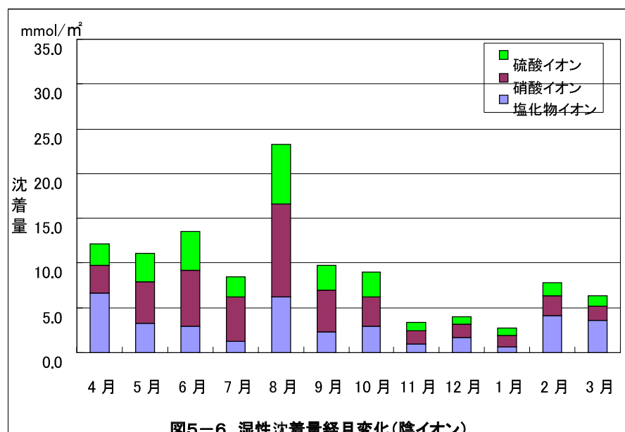
図5-6 湿性沈着量経月変化(陰イオン)
