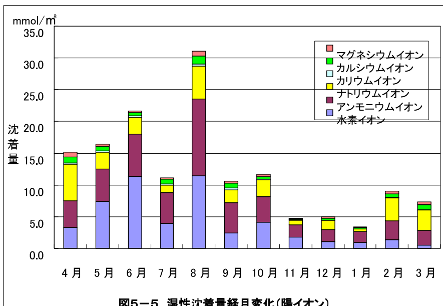
図5-5 湿性沈着量経月変化(陽イオン)
