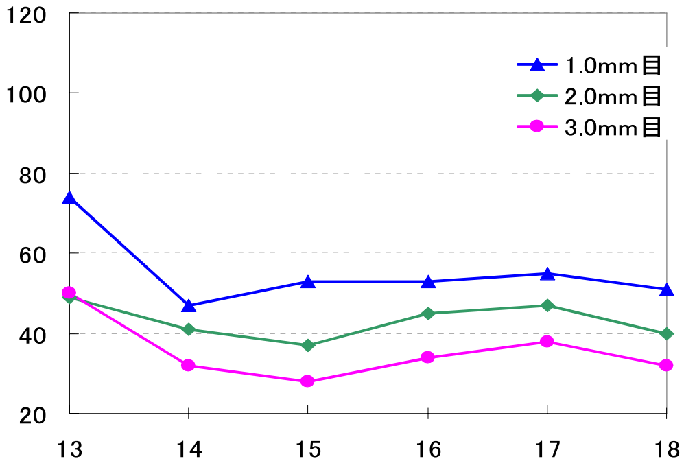
図8 初期降雨の導電率経年変化 (さいたま市役所測定局)
