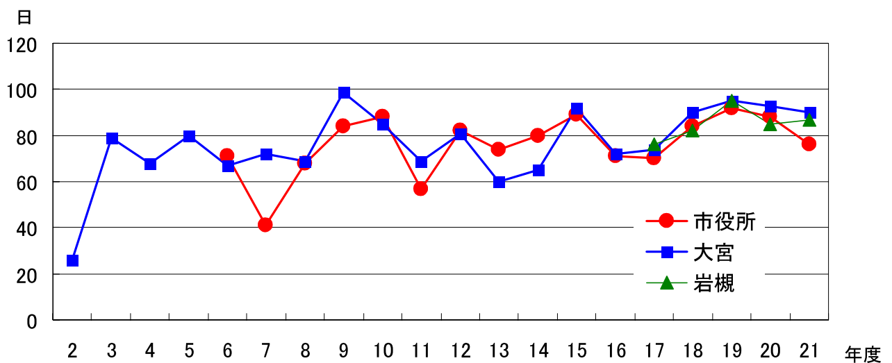
図3-1 全降雨日数の経年変化
