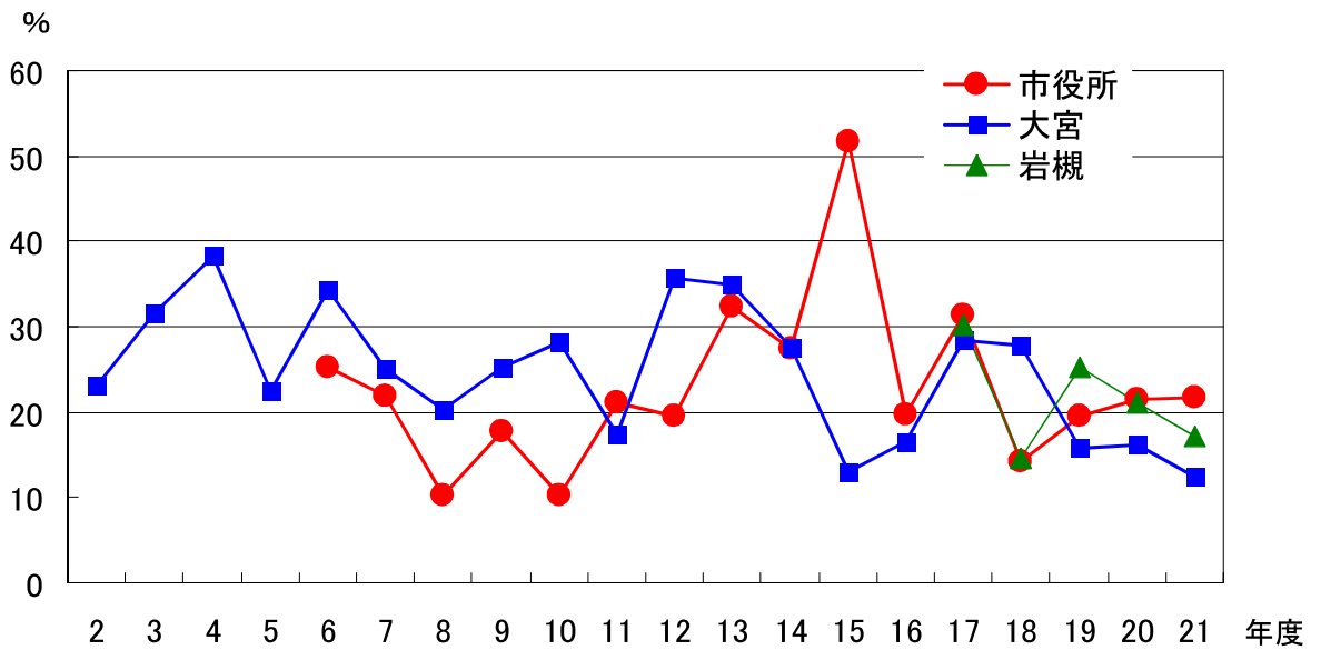
図3-2 全降雨日数に占める酸性雨(pH4.0以下)の割合の経年変化
