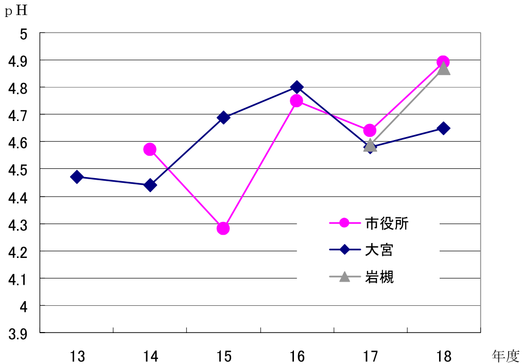
図6 年間平均 pH の経年変化
