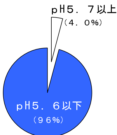
図2 全降雨に占める酸性雨の割合
