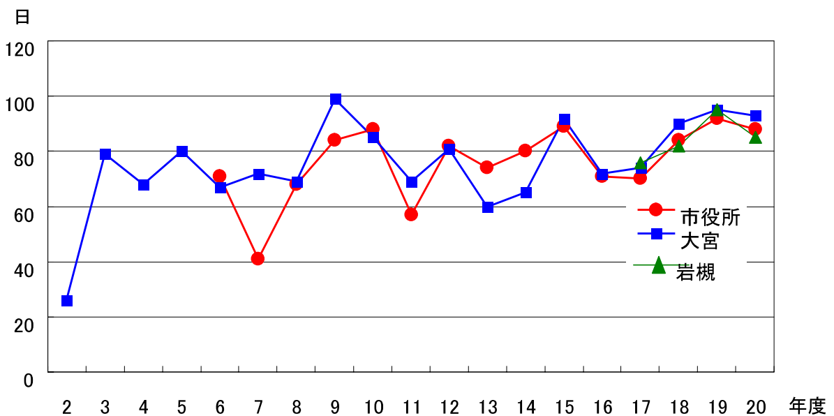
図3-1 全降雨日数の経年変化
