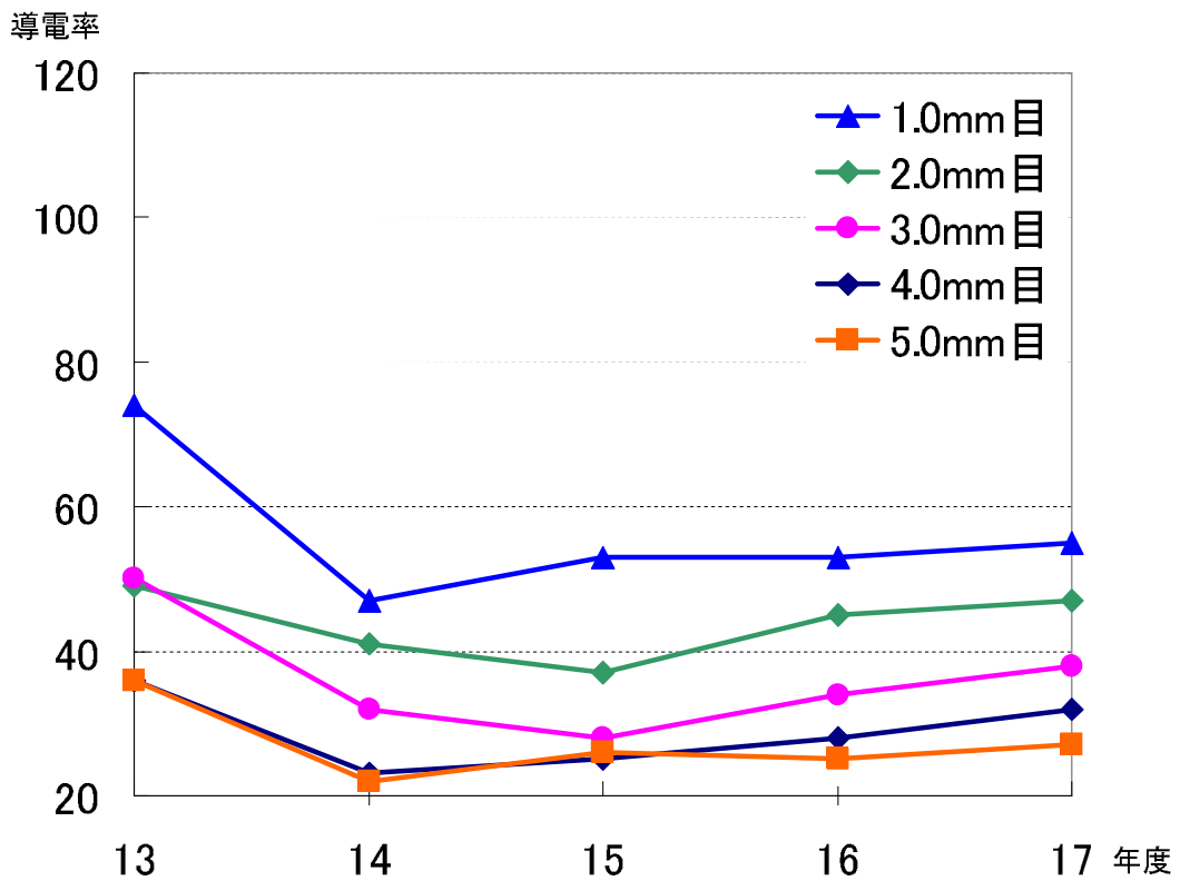
図7 初期降雨の導電率経年変化(さいたま市役所測定局)
