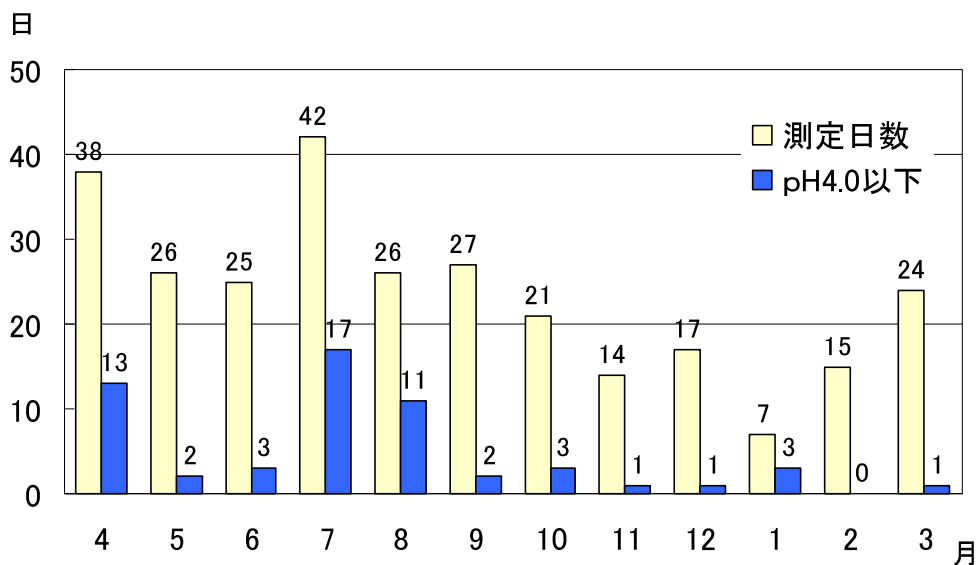
図4 pH4.0以下の降雨日数経月変化
