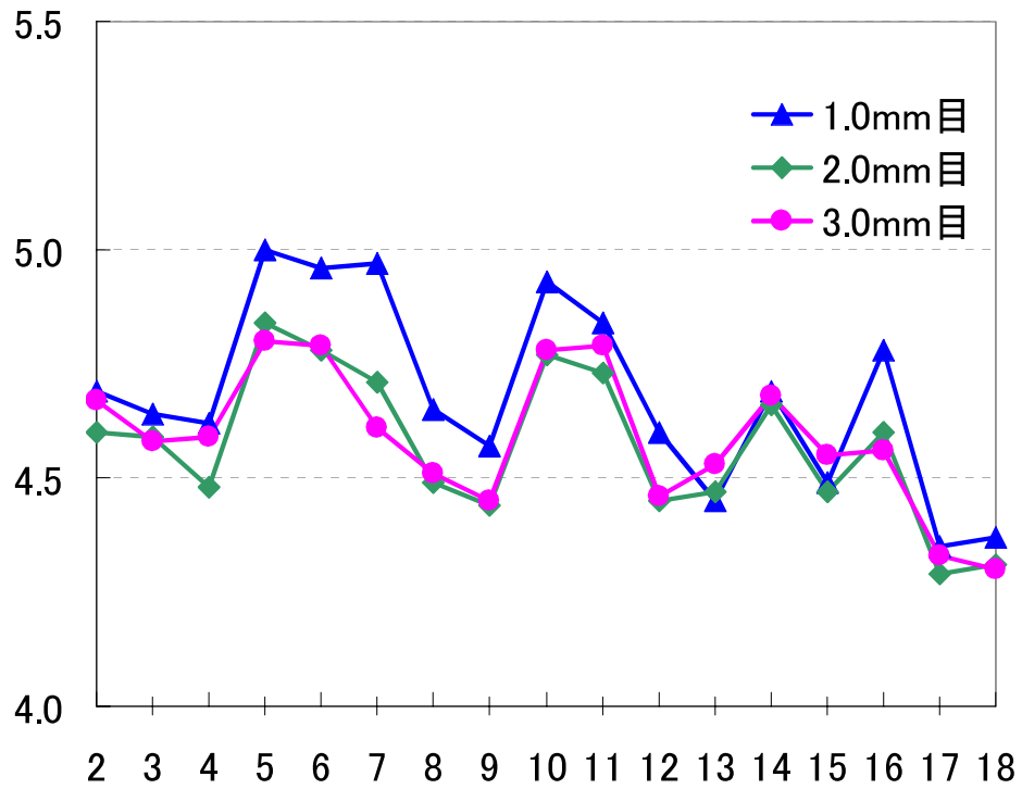
図9 初期降雨のpH経年変化 (大宮区役所)
